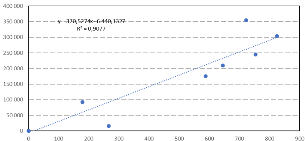
Мал. 31 – Нормалізоване вимірне споживання – існуюча ситуація
