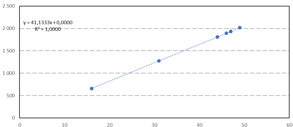
Мал. 37 – Споживання електроенергії для освітлення – після впровадження енергоефективних заходів
