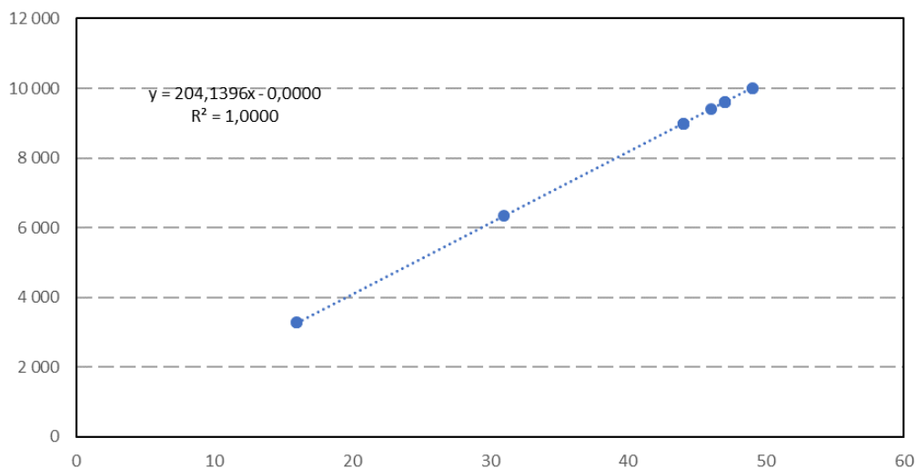
Мал. 35 – Споживання електроенергії для освітлення – існуюча ситуація
