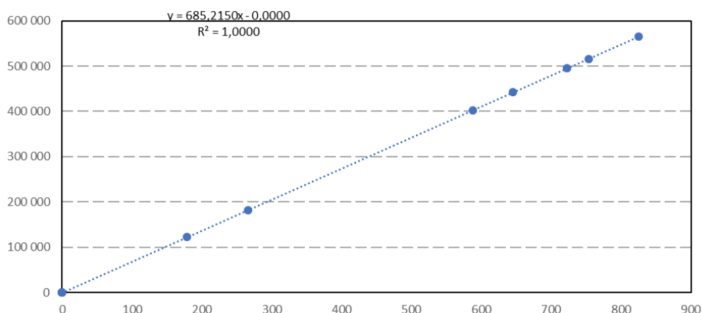
Мал. 32 – Базове споживання – існуюча ситуація
