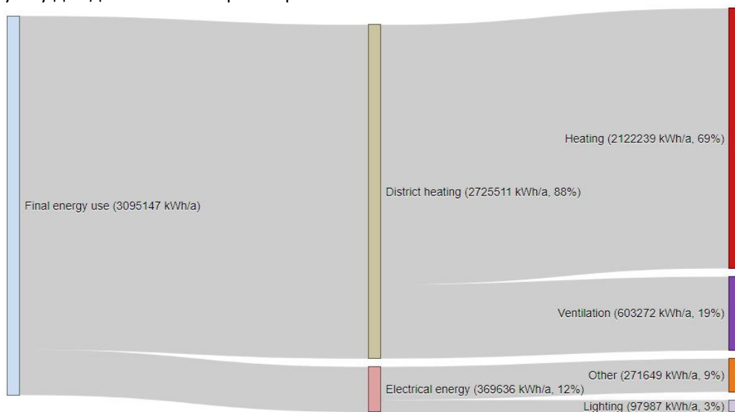
Мал. 2 – Діаграма Сенкі поточного споживання енергії
