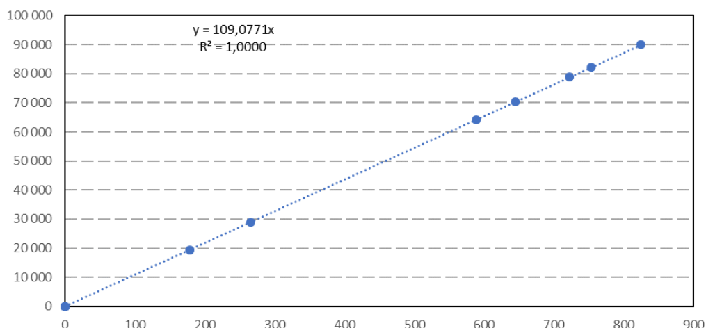
Мал. 25 – Базове споживання – після впровадження енергоефективних заходів
