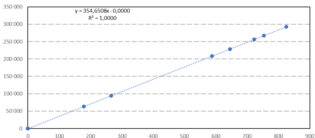
Мал. 31 – Базове споживання – існуюча ситуація
