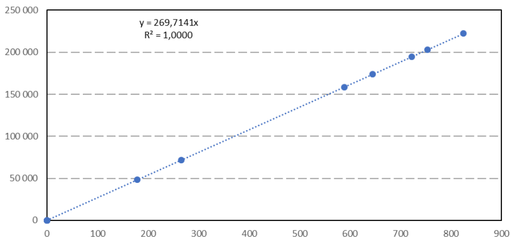
Мал. 32 – Базове споживання – після впровадження енергоефективних заходів
