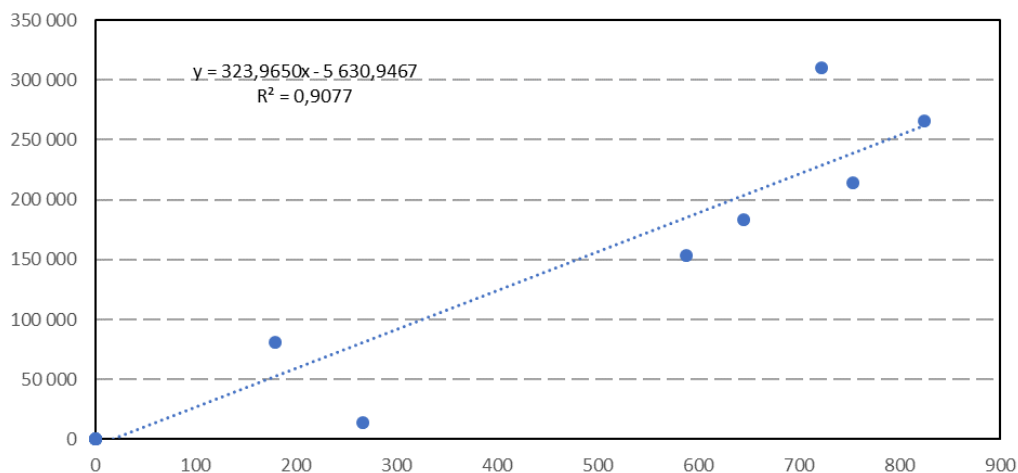
Мал. 23 – Нормалізоване вимірне споживання – існуюча ситуація
