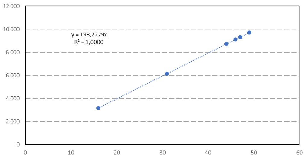
Мал. 27 – Споживання електроенергії для освітлення – існуюча ситуація
