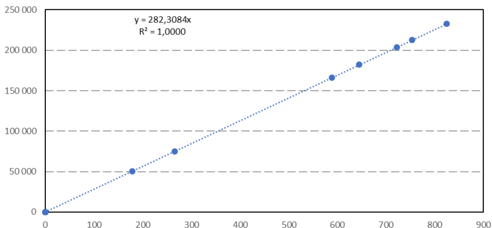
Мал. 25 – Базове споживання – після впровадження енергоефективних заходів
