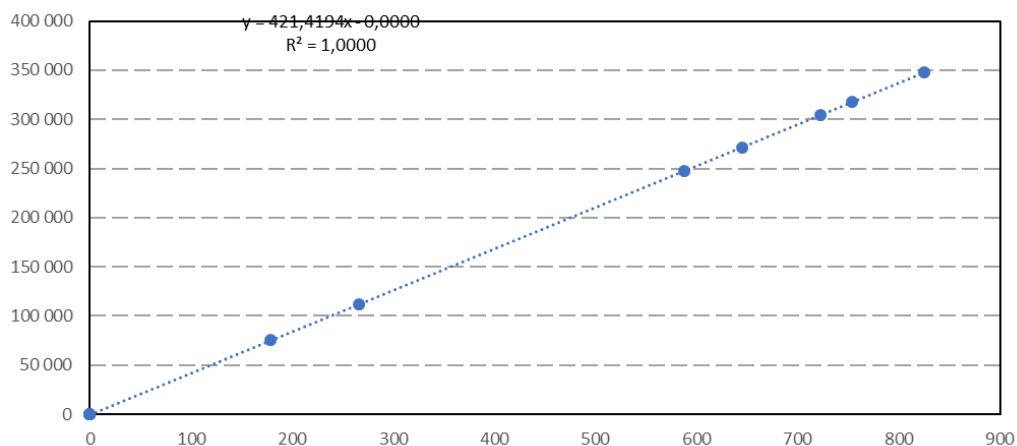
Мал. 23 – Базове споживання – існуюча ситуація
