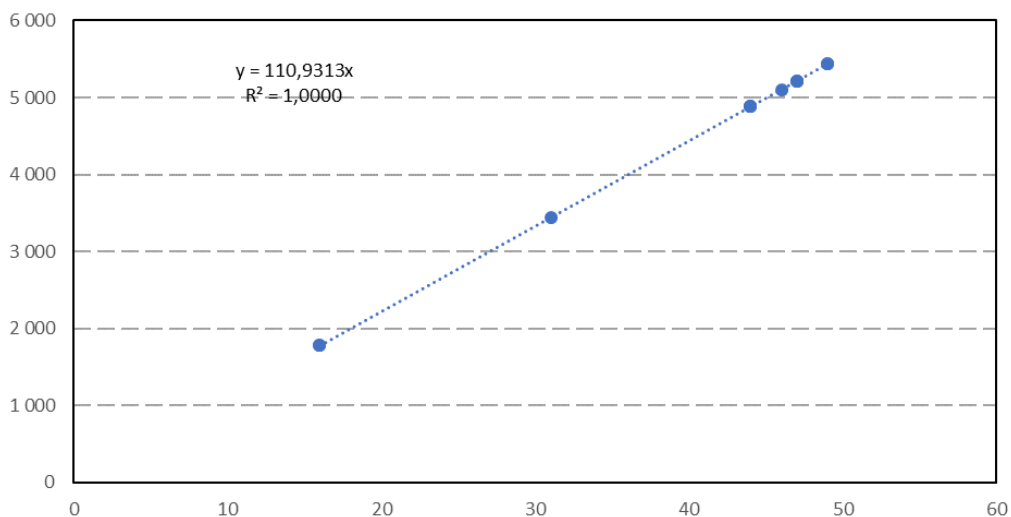
Мал. 26 – Споживання електроенергії для освітлення – існуюча ситуація
