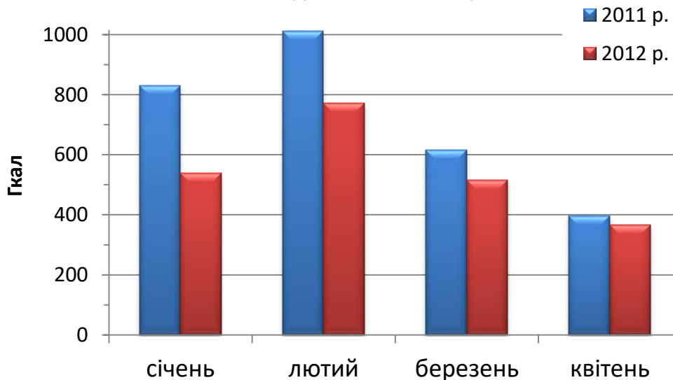
Споживання тепла гуртожитками СумДУ
